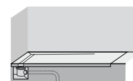
Instalación encastrada Sunken into floor
