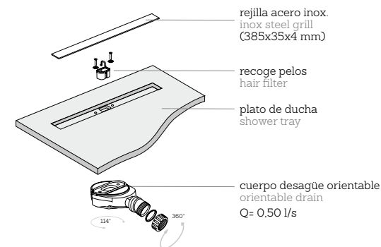
Instalación sobre el suelo Flat to floor
